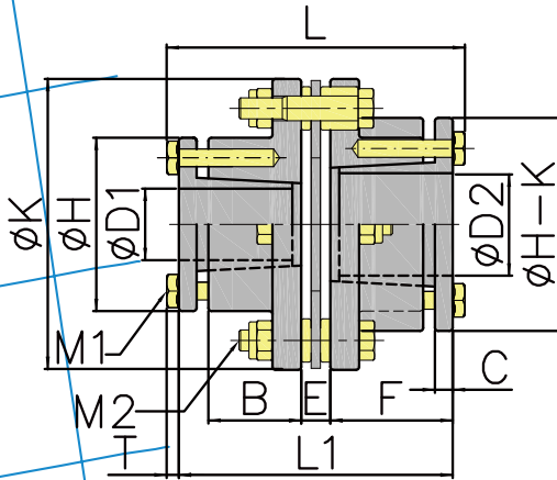
材質: S45C
